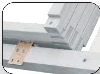
Montering på lægter
